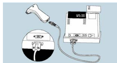
Lesestiftemulation
